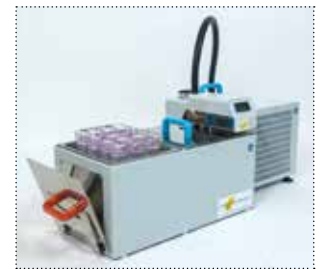
Pasteurierer T30
